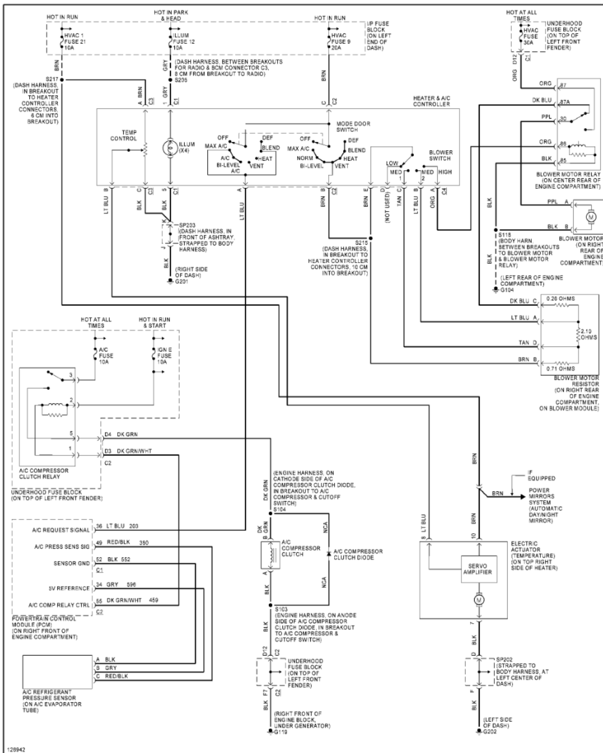
Fig. 2: 2.2L VIN 4, Manual A/C Circuit
