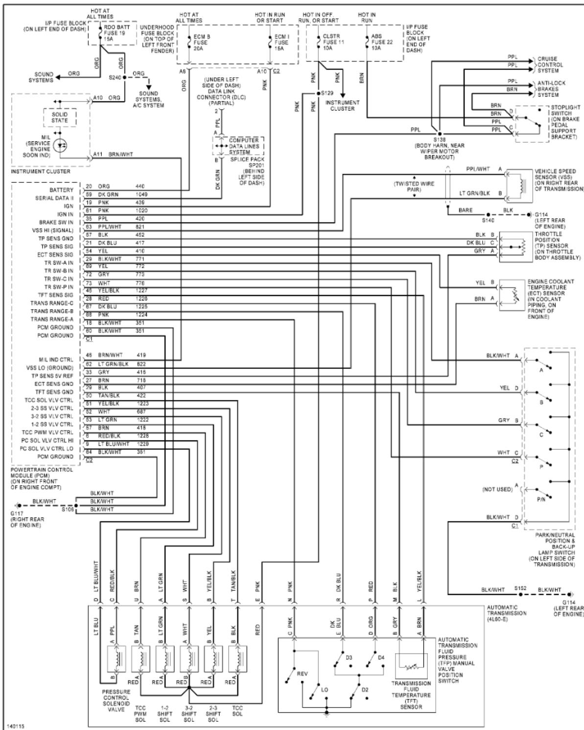
Fig. 59: 2.2L VIN 5, A/T Circuit, 4L60-E
