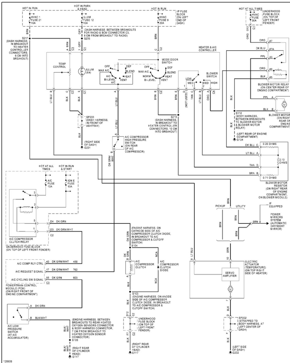
Fig. 5: 4.3L VIN W, Manual A/C Circuit
