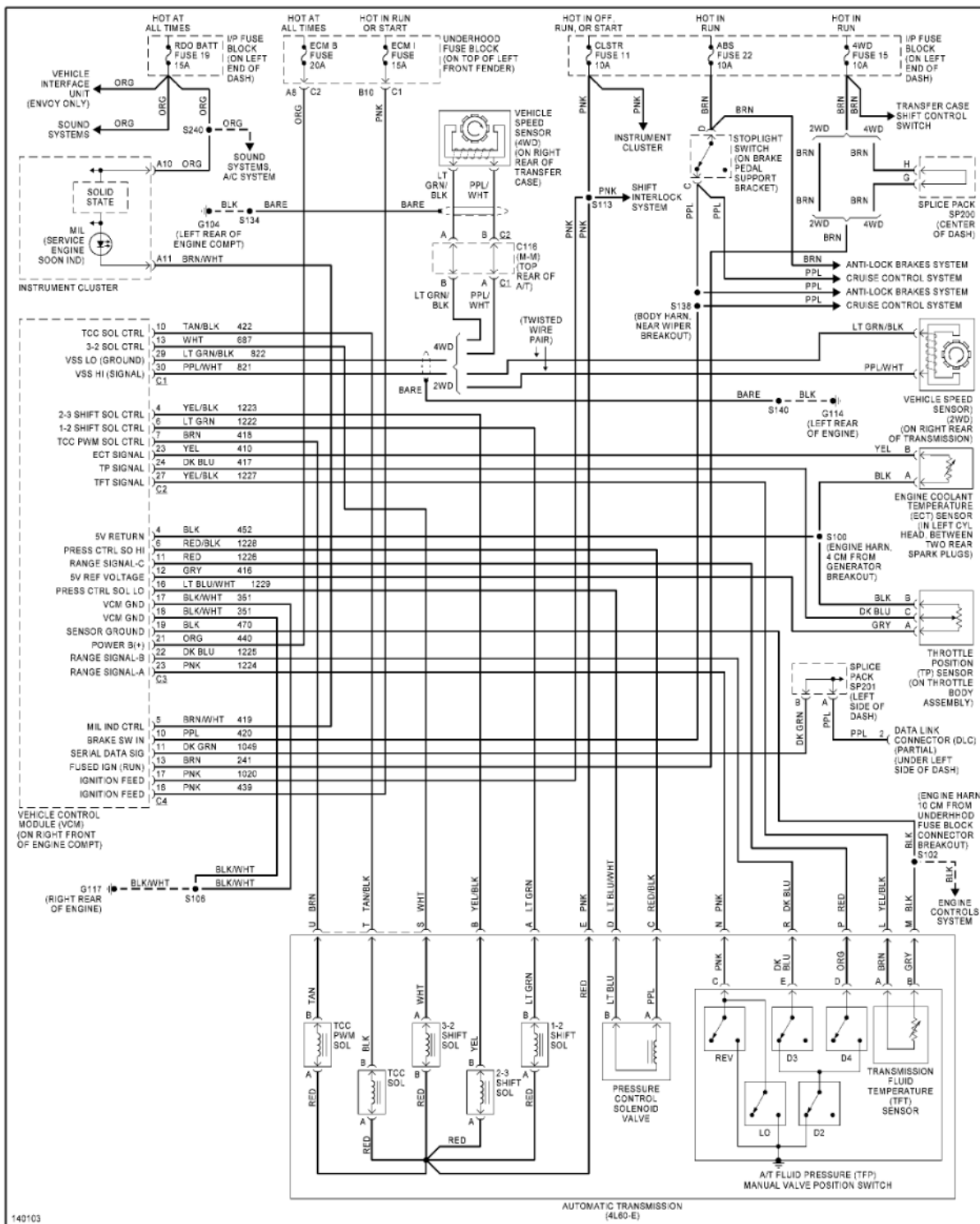
Fig. 61: 4.3L VIN W, A/T Circuit, 4L60-E
