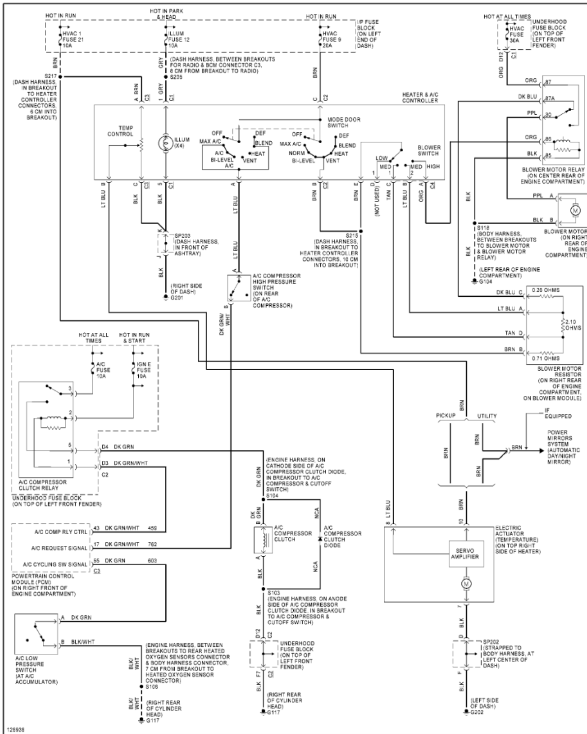
Fig. 7: 4.3L VIN X, Manual A/C Circuit
