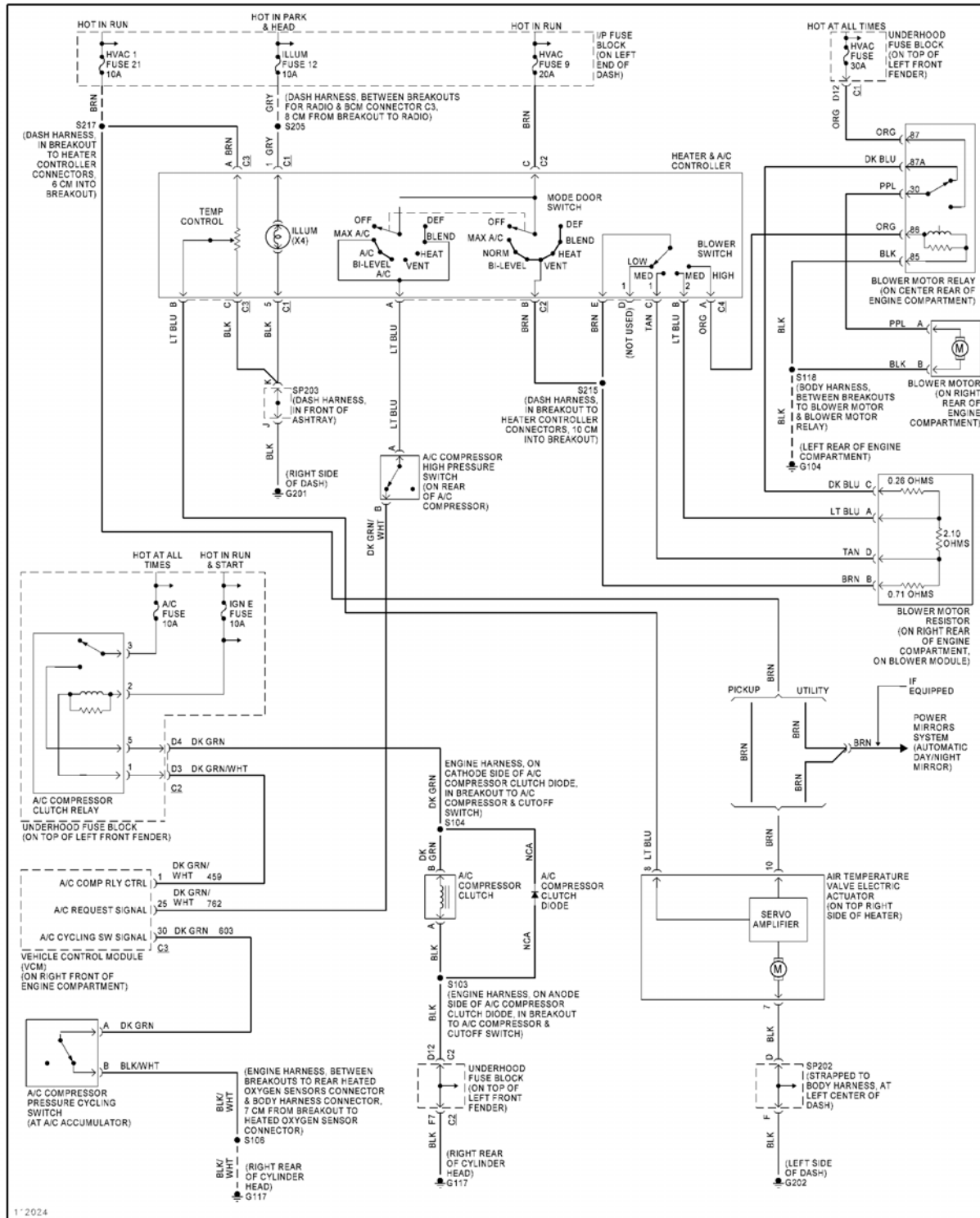
Fig. 7: 43L VIN X, Manual A/C Circuit
