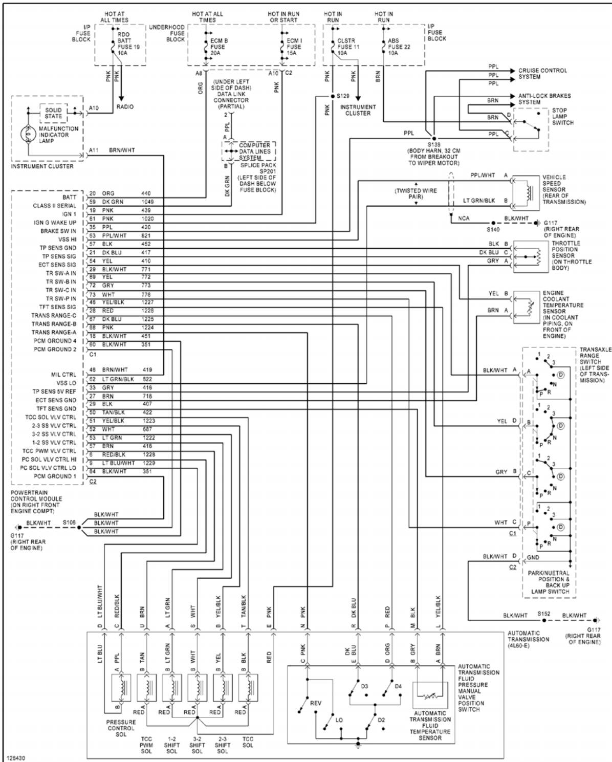
Fig. 53: 2.2L VIN 4, A/T Circuit, 4L60-E
