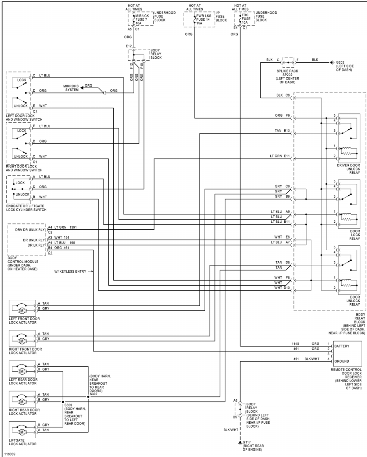
Fig. 43: Power Door Lock Circuit
