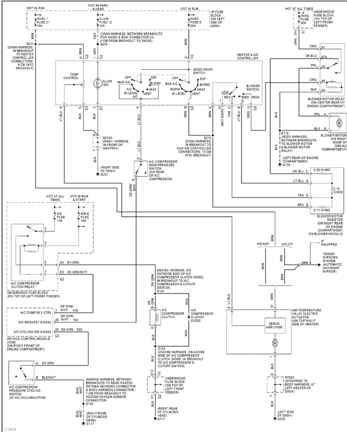
Fig. 5: 43L VIN W, Manual A/C Circuit
