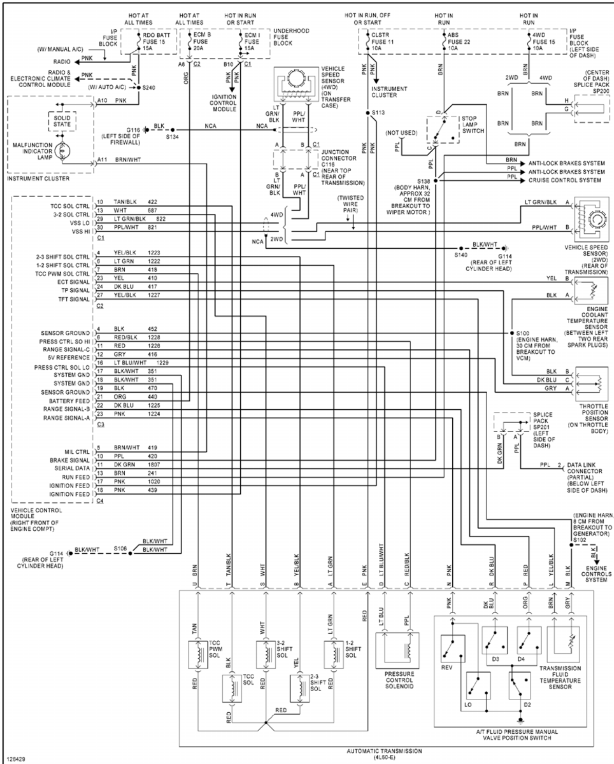
Fig. 57: 4.3L VIN X, A/T Circuit, 4L60-E
