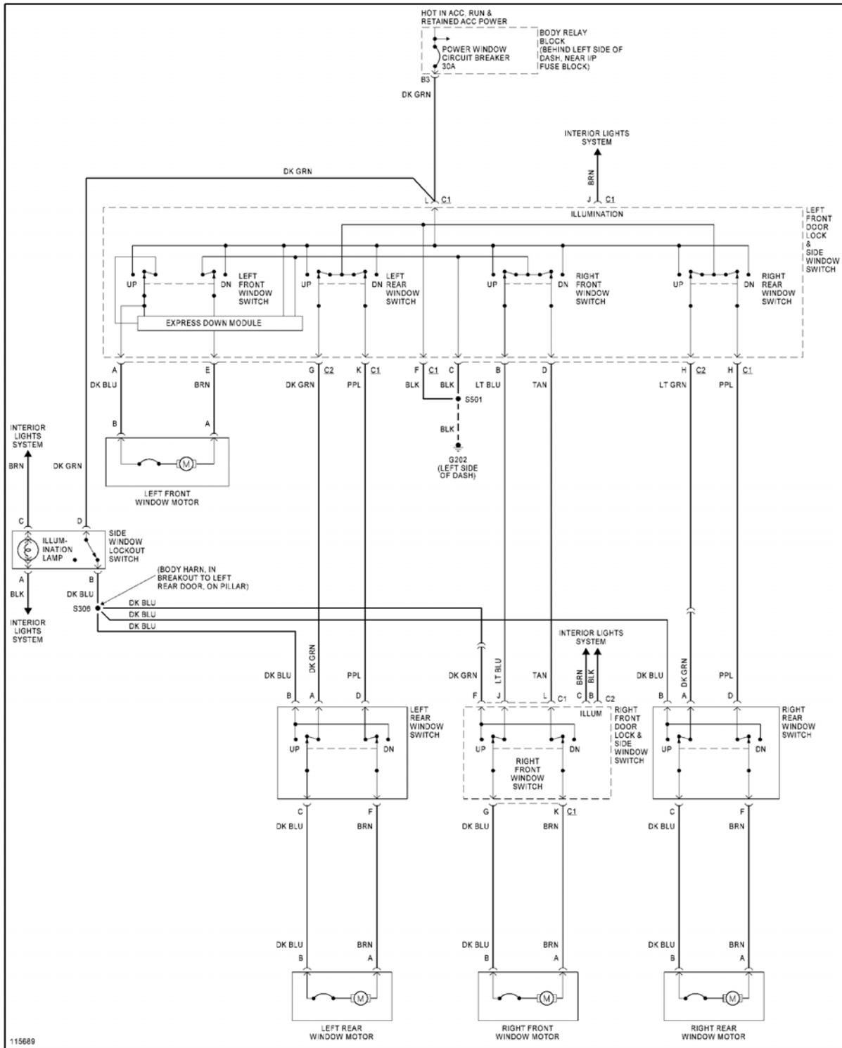
Fig. 46: Power Window Circuit, 4 Door
