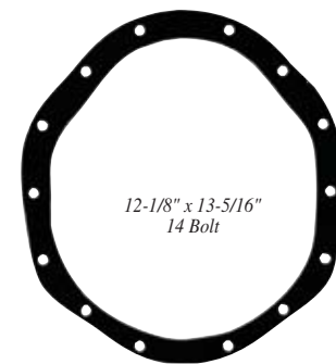
GM-14 Bolt-9.5" Ring Gear
