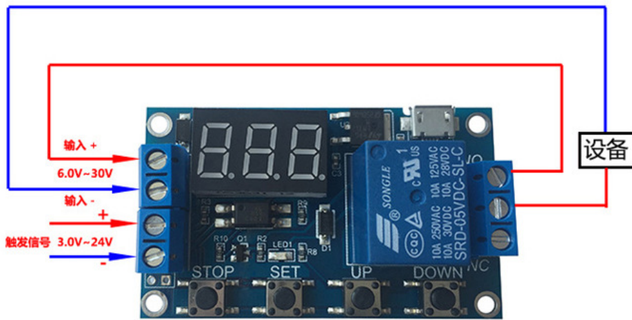
共用一个电源的接线图
