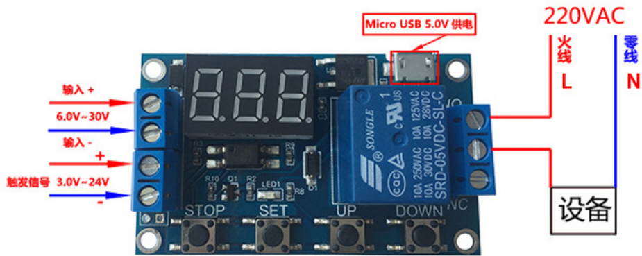
弱电控制强电接线图
